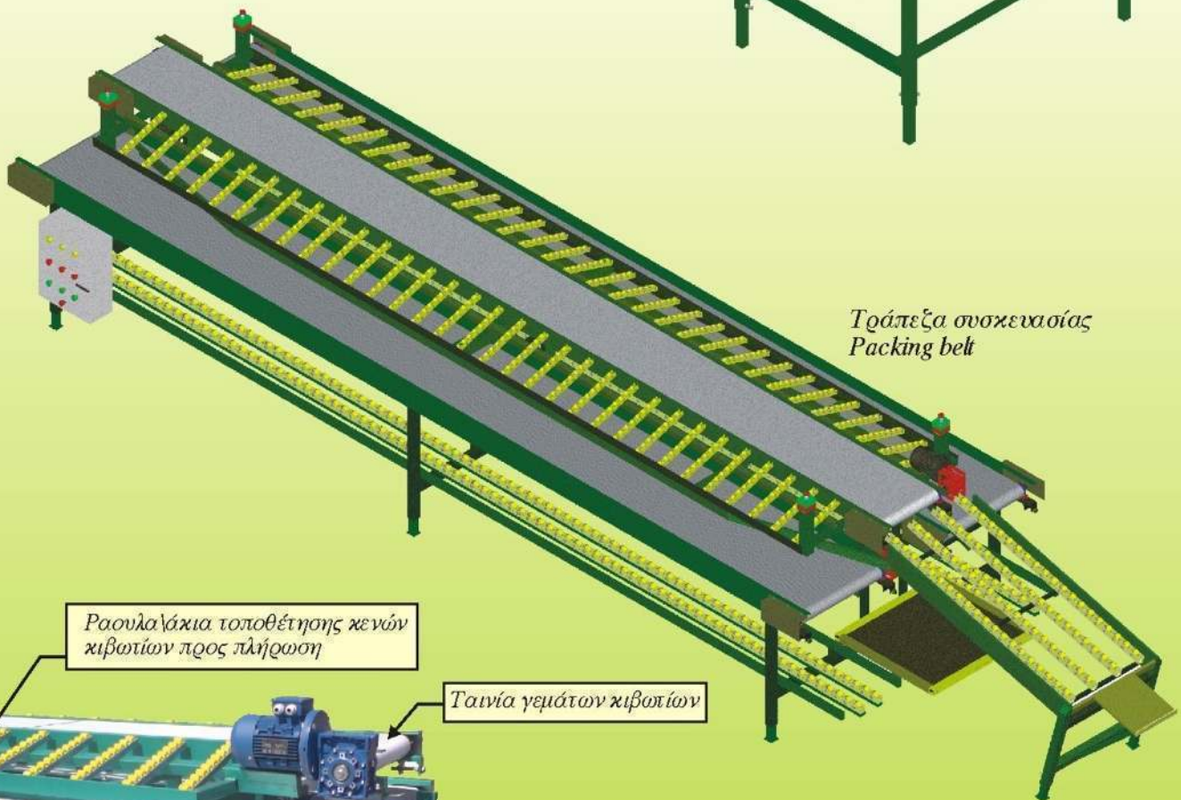
Μεταφορική ταινία φρούτων Conveyor belt
