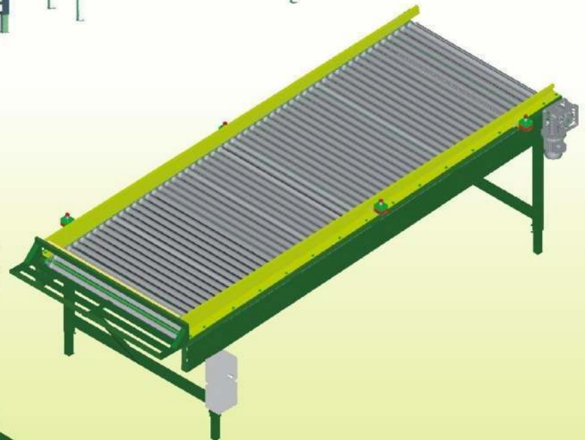
Ανεβαστήριο - Τράπεζα προδιαλογής με επενδυμένα ρόουλα Elevator - Pre-sorting table with facing rolls
